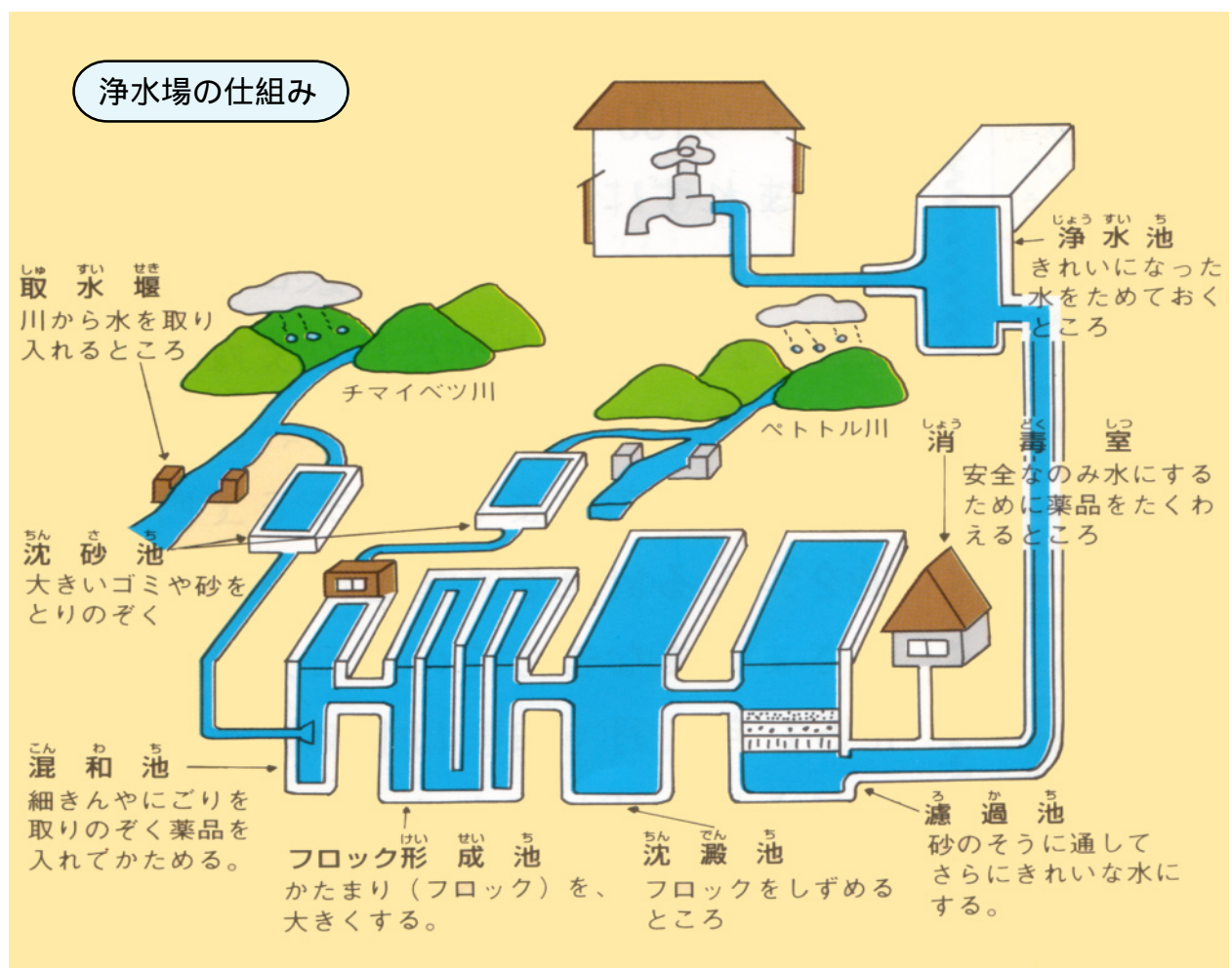
浄水場のなかのようす
